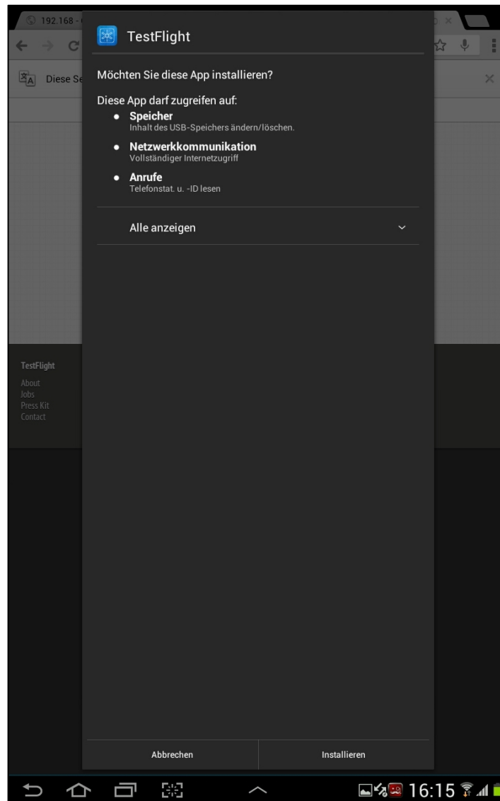
Abbildung 7: Installieren anklicken
