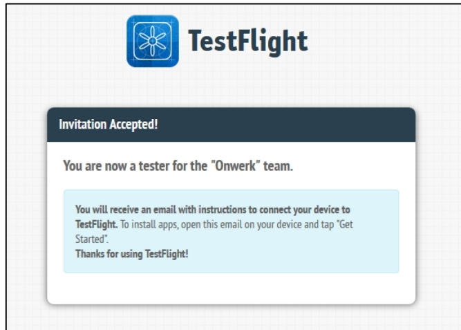
Abbildung 3: Anmeldebestätigung
