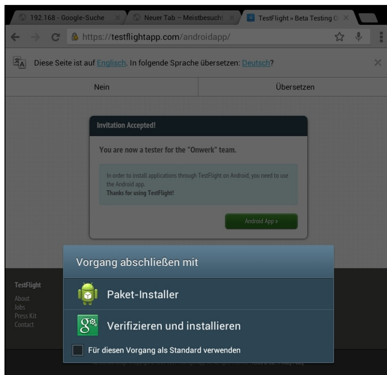
Abbildung 6: Paket-Installer auswählen
